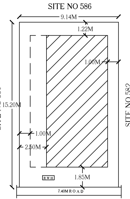
SITE PLAN 1:200
